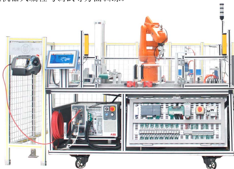
图 1 赛项平台（工业机器人与智能视觉应用）
